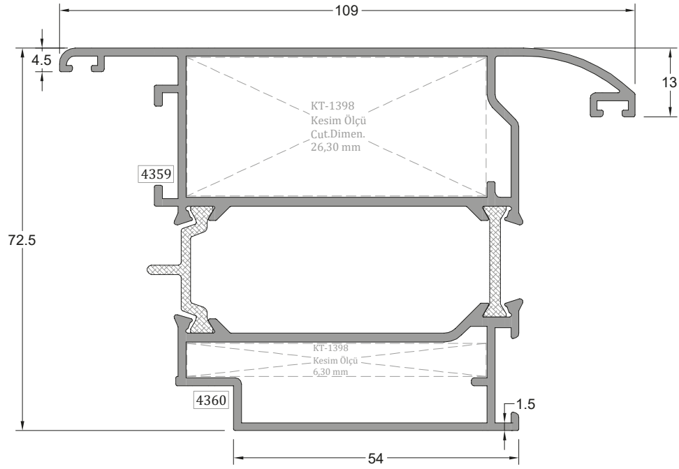
Dışa Açılır Kanat Profili OUTWARD OPENING SASH PROFILE
