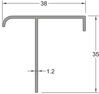
T Bağlantı Profili T CONNECTION PROFILE
