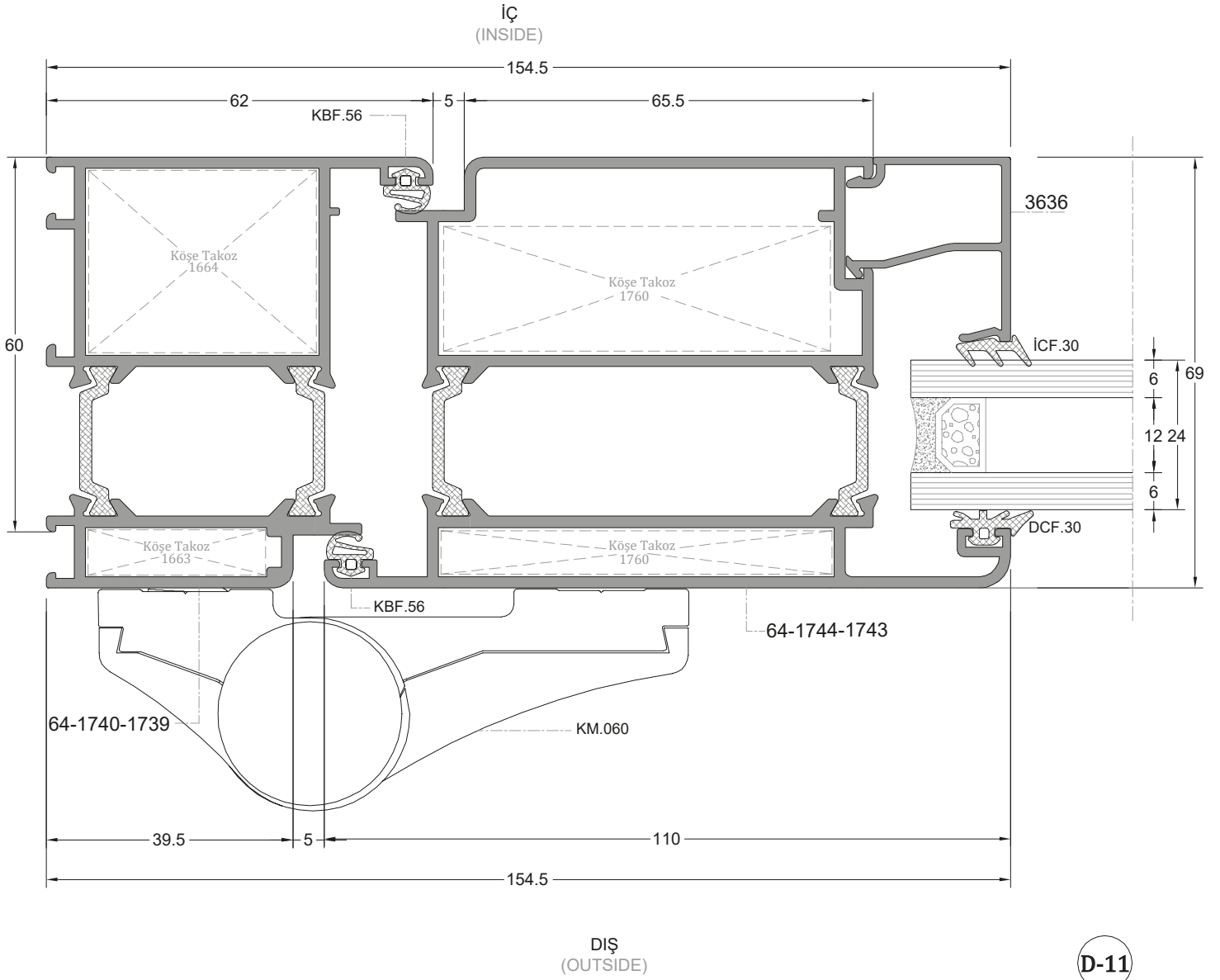
HEMYÜZ DIŞA AÇILIR KAPI DETAY
