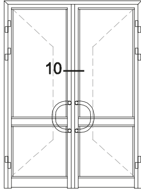
HEMYÜZ İÇE AÇILIR KAPI DETAY
