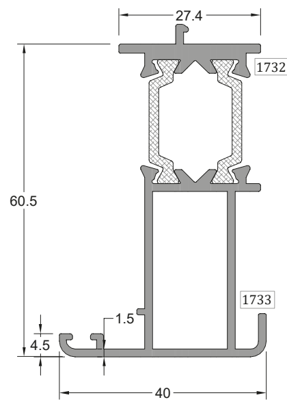
★Hemyüz Dışa Açılır Adaptör Profili OUTWARD OPENING ADAPTER PROFILE
