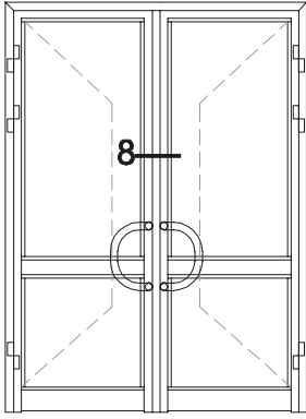
BİNİLİ DIŞA AÇILIR KAPI DETAY
