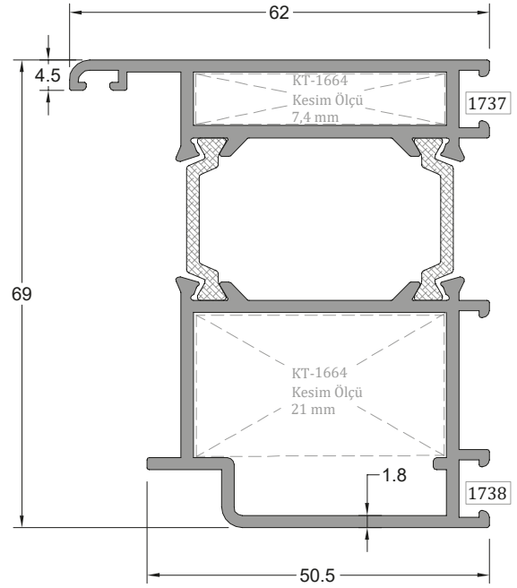
★Hemyüz İçe Açılır Kasa Profili INWARD OPENING FRAME PROFILE
