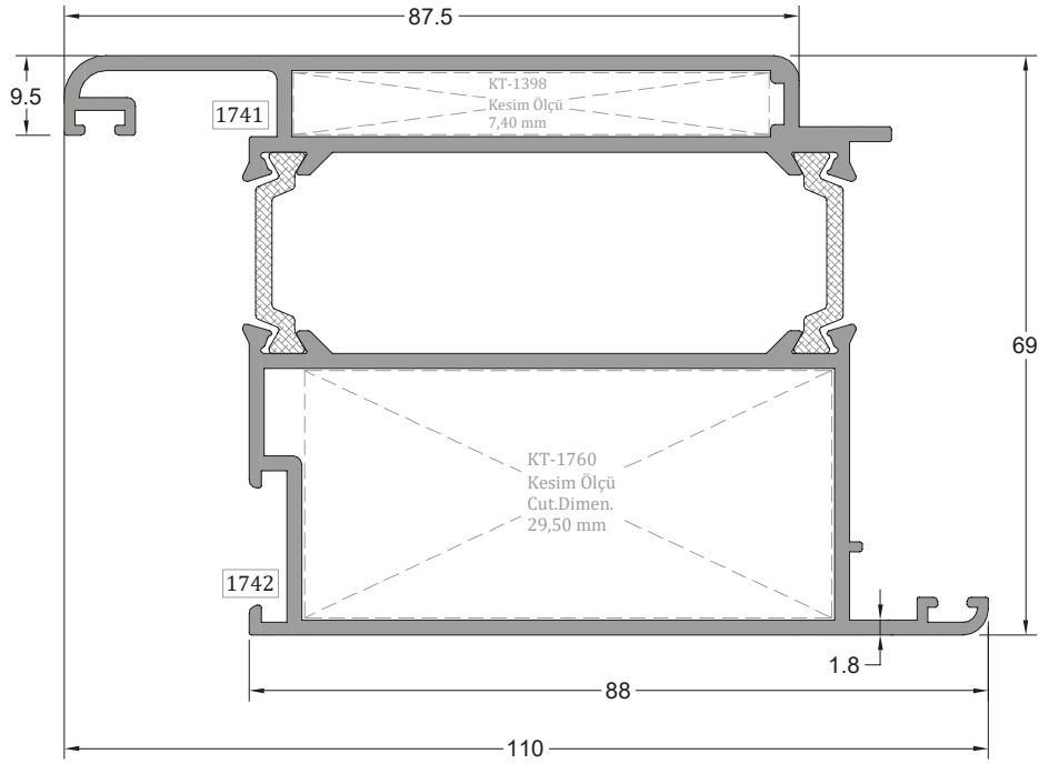
★ Hemyüz İçe Açılır Kapı Kanat Profili INWARD OPENING SASH PROFILE
