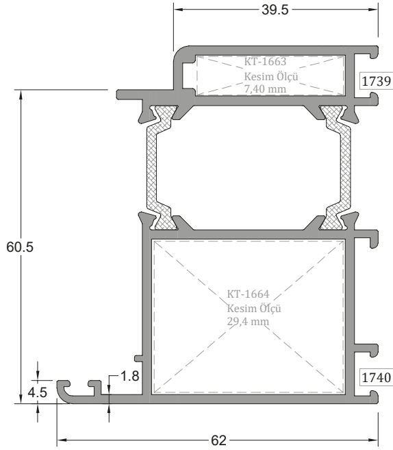
★Hemyüz Dışa Açılır Kasa Profili OUTWARD OPENING FRAME PROFILE
